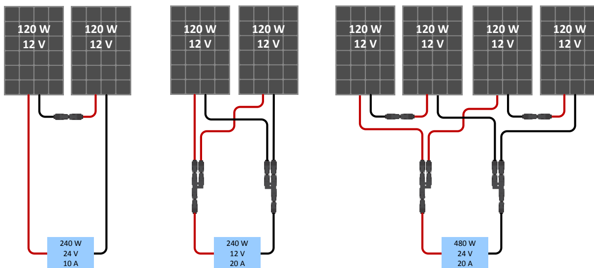
Voorbeelden van serie-, parallele- en serie / parallelle zonnepanelen.
